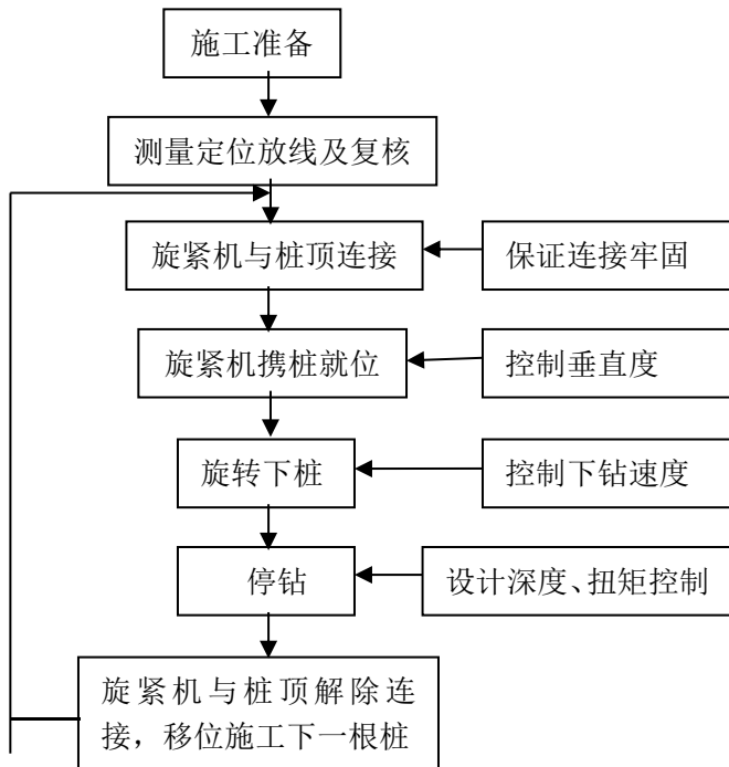
图 5.2.2 桩施工流程框图
